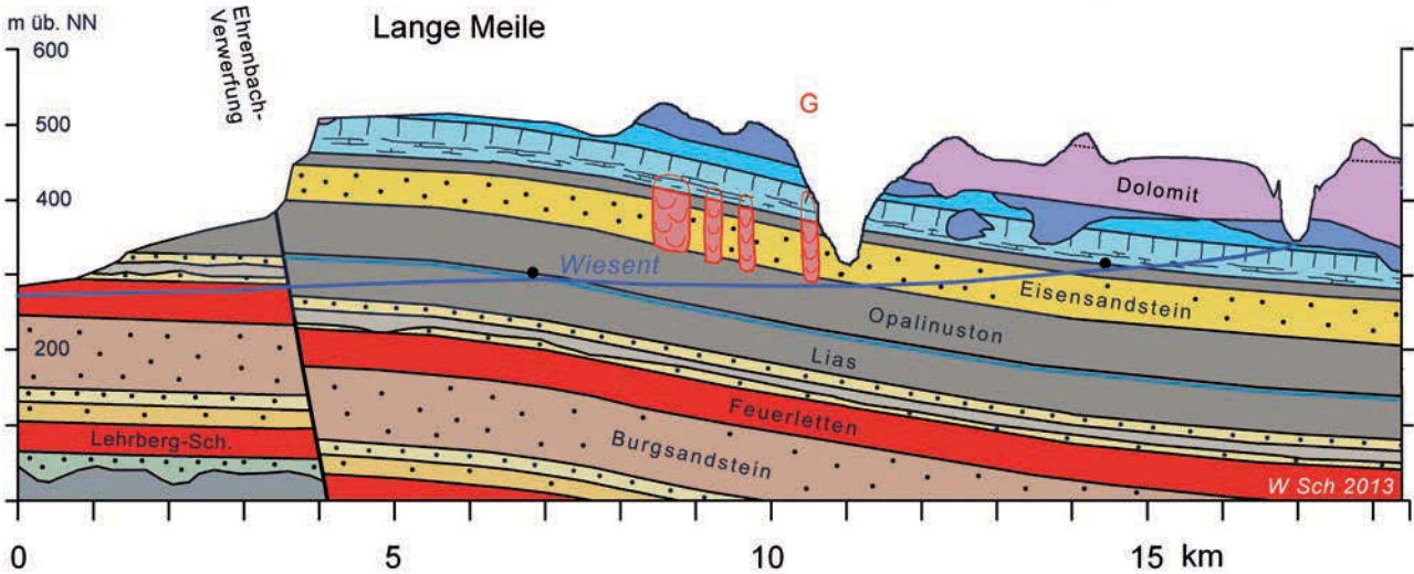
Bild 2 Schnitt durch die Fränkische Schweiz von Forchheim nach Doos mit Eintrag des Wiesentlaufes (blaue Linie). G = Gasseldorfer Berggrutsch.
