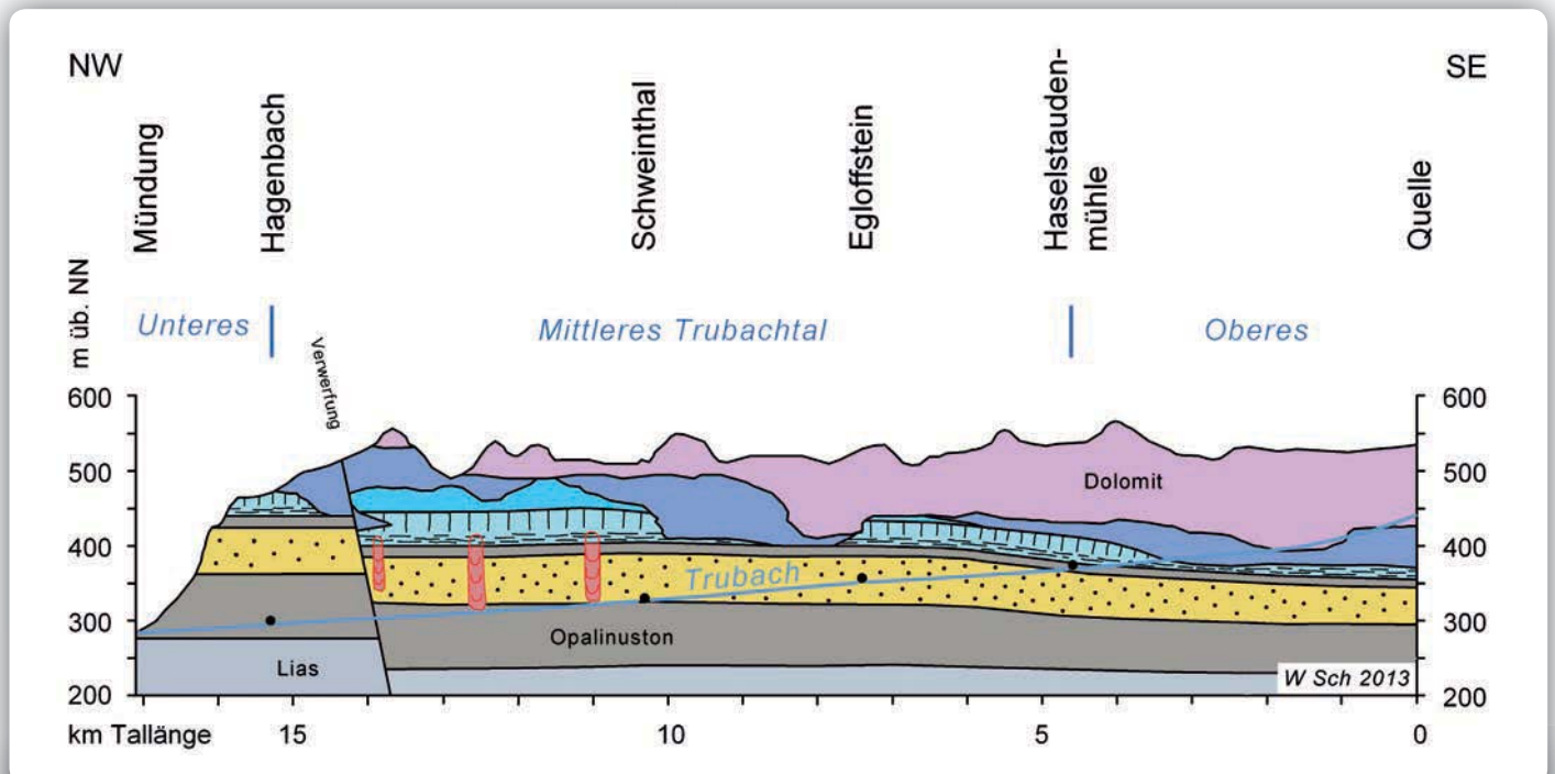
Bild ❶ Längsschnitt entlang dem Trubachtal von der Quelle (rechts) zur Mündung in die Wiesent (links). Die Trubach ist mit blauer Linie eingetragen. Die Legende ist unter Bild ❷.
